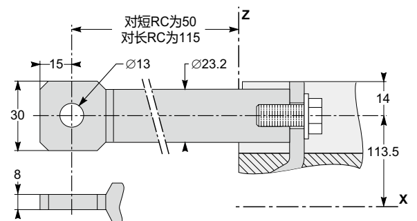
后连接端子 (RC)
