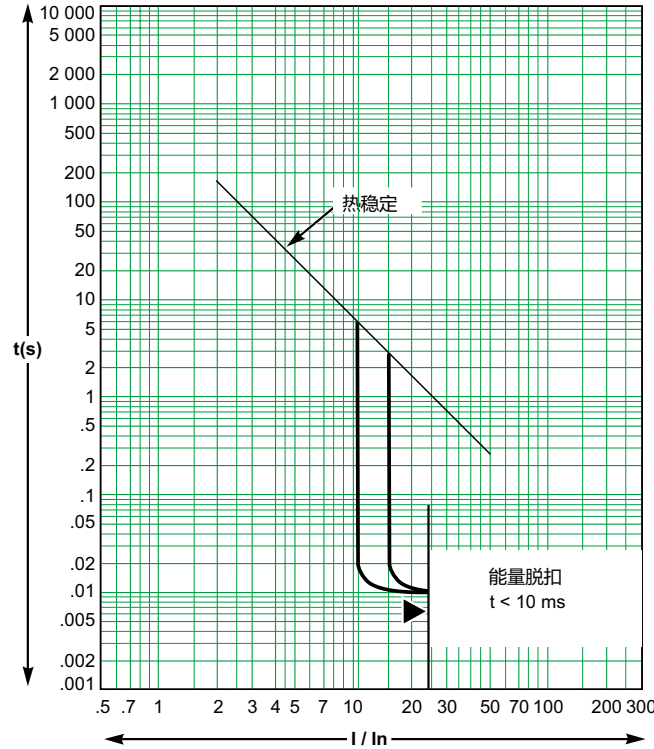
电子脱扣器 500 A
