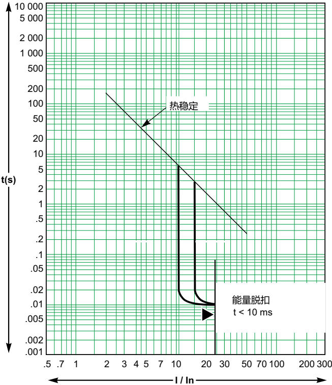
电磁脱扣器 320 A
